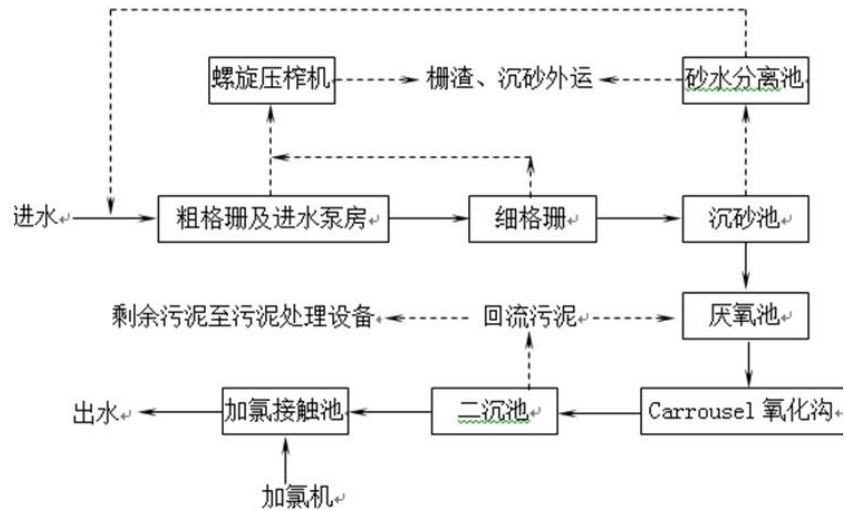
图 4-1 白荡水质净化厂废水处理工艺流程图
