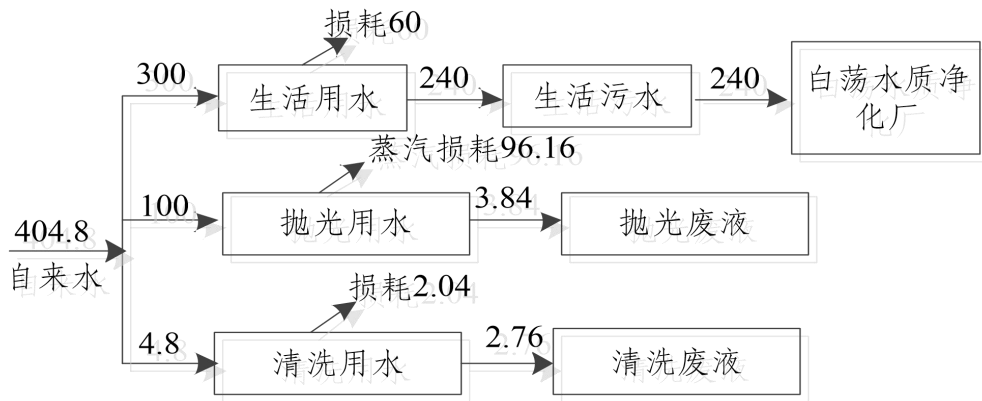
图 2-1 改建项目水平衡图 (m 3 /a)
