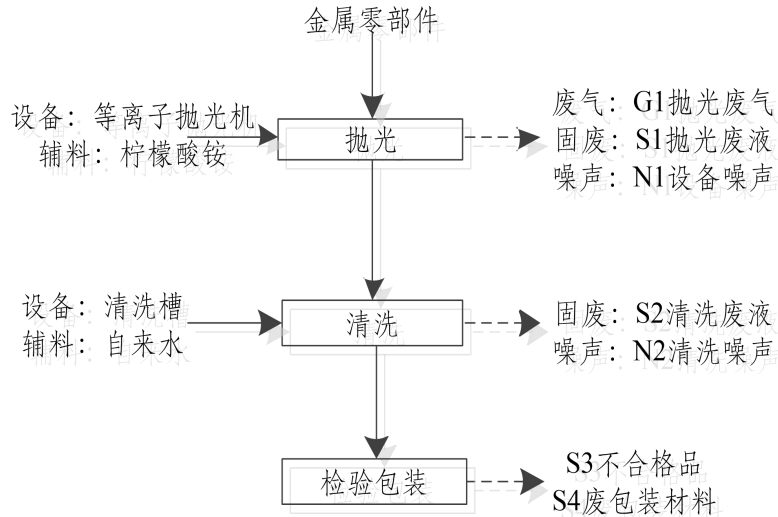
图 2-2 金属零部件加工流程图
