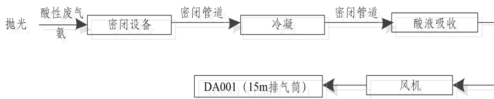
图 4-1 项目废气收集、处理系统图
