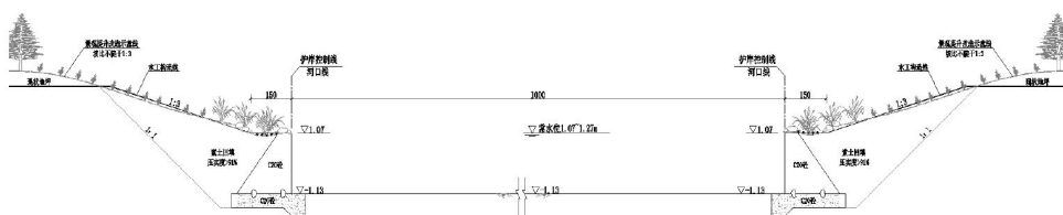
图 2-7 西浜河道断面图
