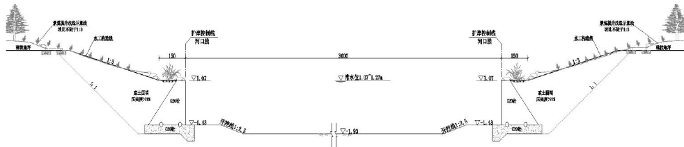
图 2-5 中桥港河道断面图
