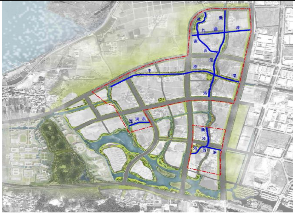
图 2-1 本项目河道平面图
