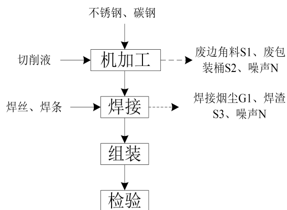
图5-1 生产工艺流程及产污环节图
