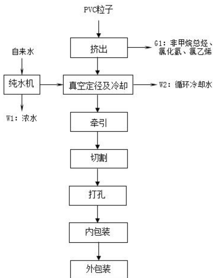
图 2-1 项目工艺流程图及产污环节
