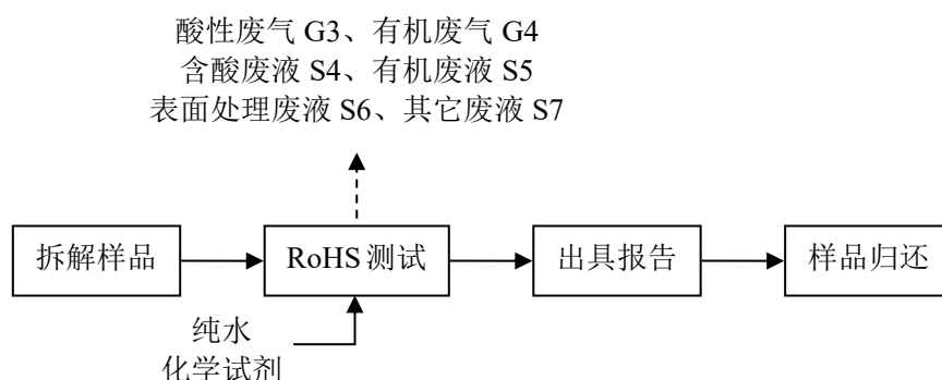
图 5-5 RoHS 检测工艺流程图
