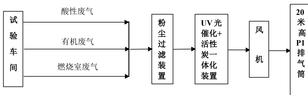
图 5-7 P1 排气筒废气排放流程
