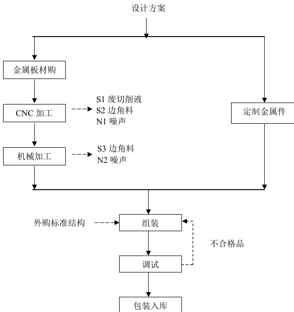
图 5-1 工艺流程图
