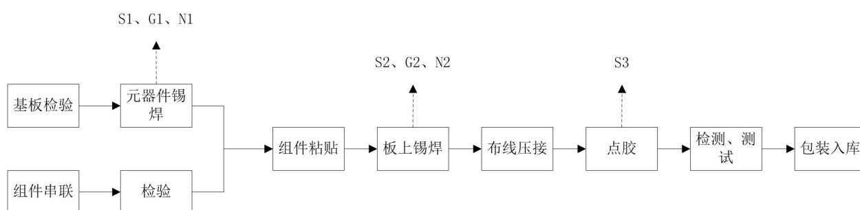
图 5-1 工艺流程图
