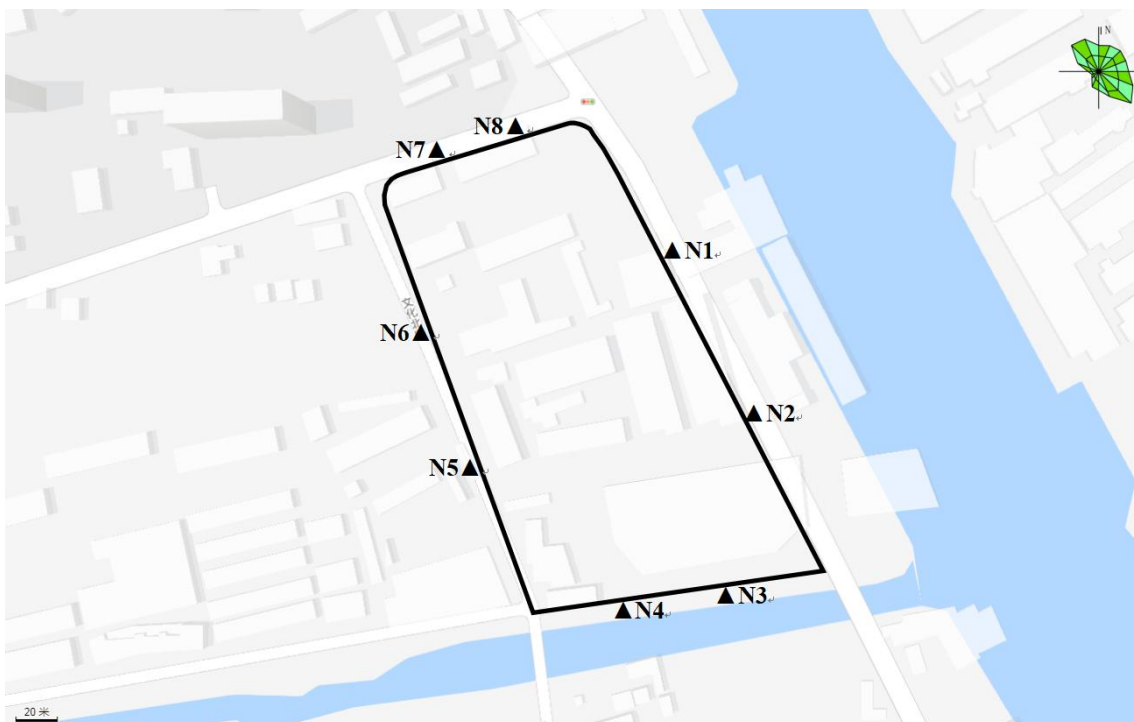
图 7.4-1 项目环境监测点位布置图
