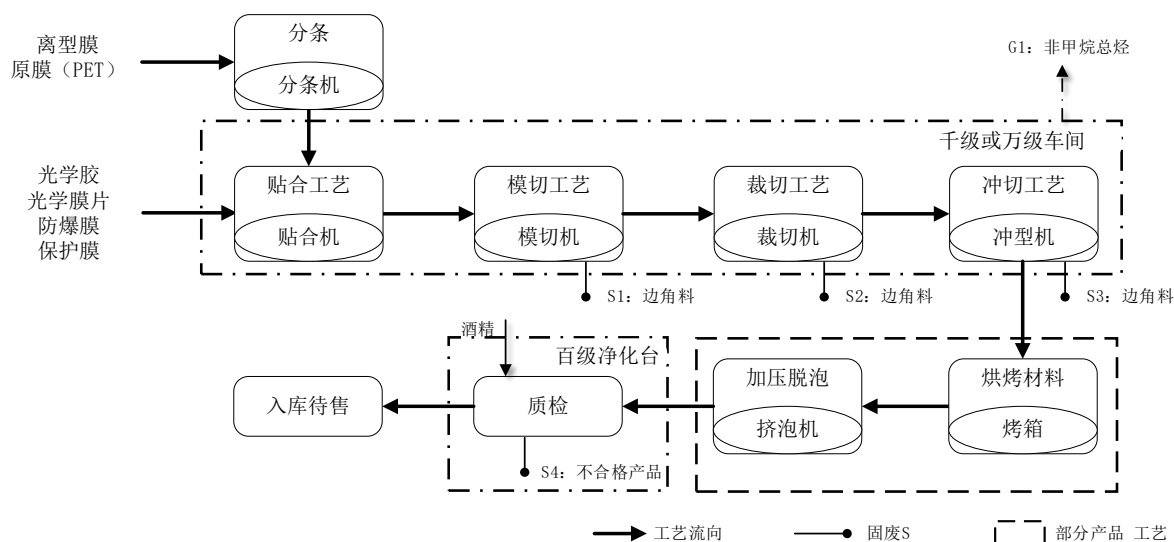
图 5-1 项目生产工艺流程及产污节点图
