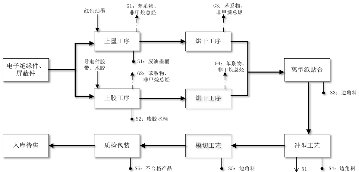
图 1-1 原有项目生产工艺流程
