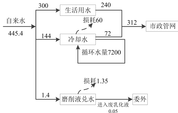
图5.3-1 项目水平衡图
