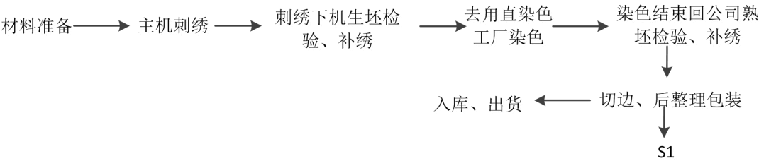
图 1-1 刺绣花边的生产工艺流程图
