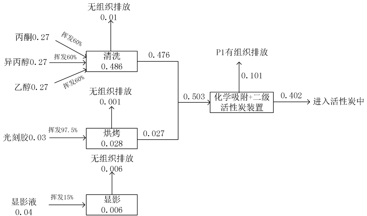
图 3.7-2 本项目 VOC 物料平衡图（单位 t/a）
