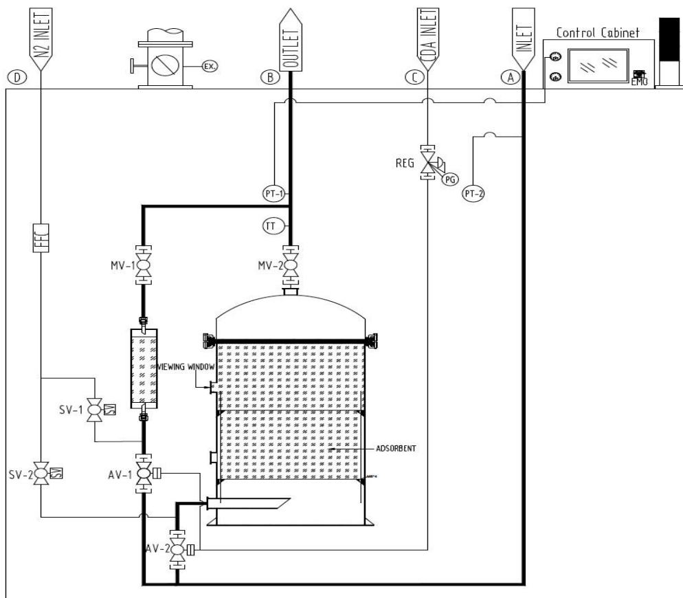
图 6.2-1 化学吸附装置
