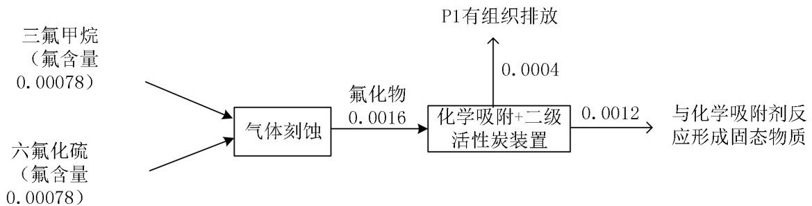
图 3.7-3 本项目氟元素平衡图（单位 t/a）
